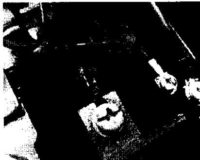
Circuito de tensión QUEMADO (Puente de neutro y conductor)
