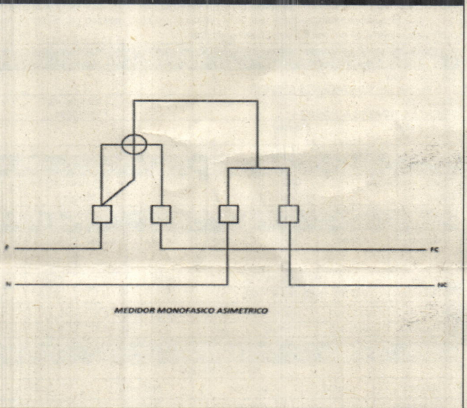
DIAGRAMA UNIFILAR DESPUES DE LA REVISION
