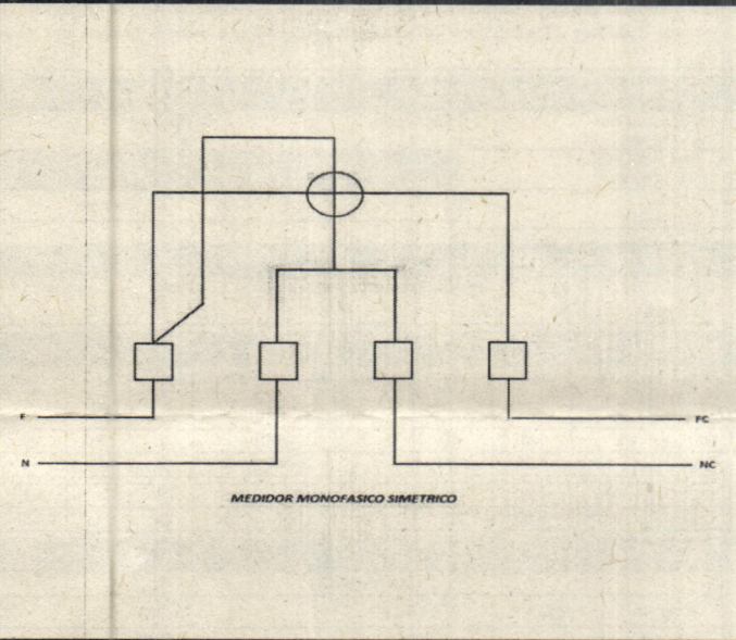
DIAGRAMA UNIFILAR ANTES DE LA REVISION
